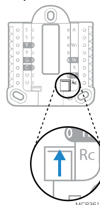
Onglet coulissant R/Rc
